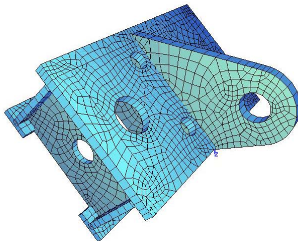
Statisches Modell – Einbauteil (Tragseilverankerung)
