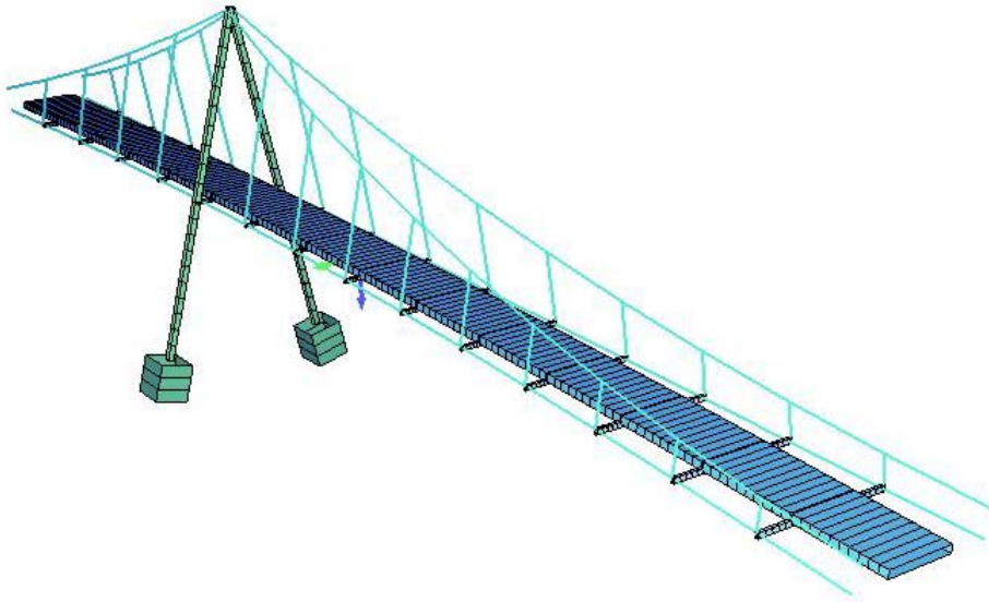
Statisches Modell - Tragwerk
