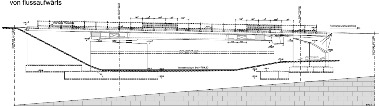
Ansicht Lippbauerbrücke
