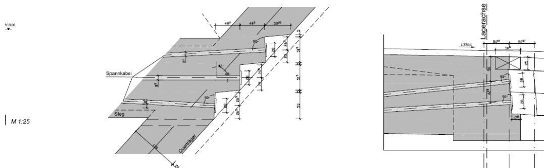
Anordnung der Spannglieder - Endquerträger
