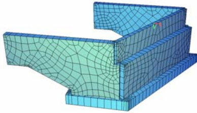
Statisches Modell Widerlager
