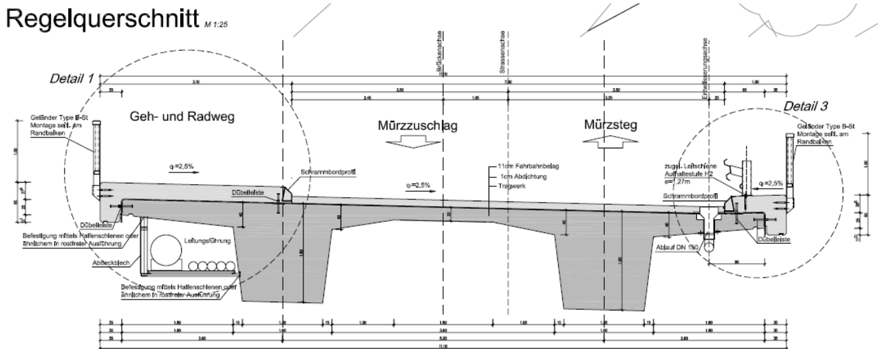
Regelquerschnitt
