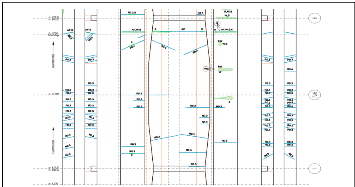
Ansichten Tragwerk Platte und Träger mit Fehlstellen des schlaff bewehrten Teiles
